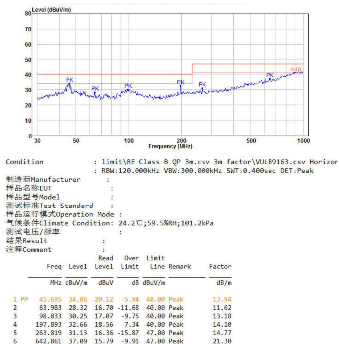
图 5-7 辐射测试垂直方向
