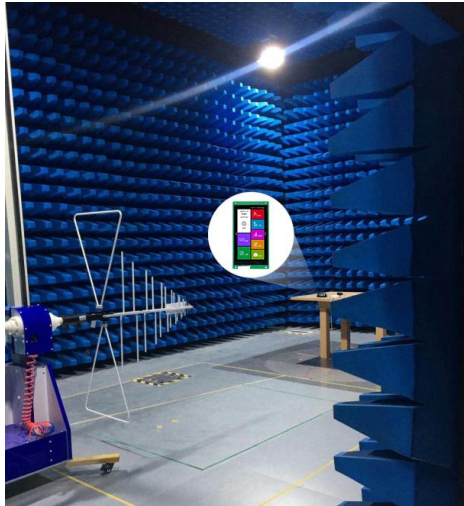
图 5-5 辐射测试图
