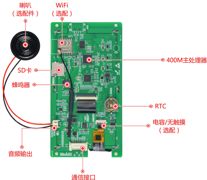
图 1-3 硬件配置图
