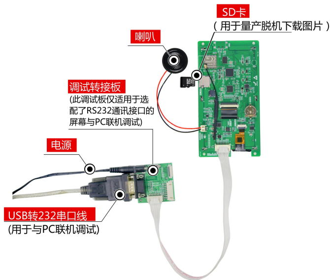
图 1-4 调试工具图
