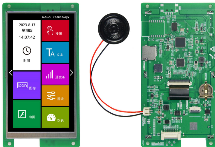
图 1-2 5.5 寸无触摸参考图
